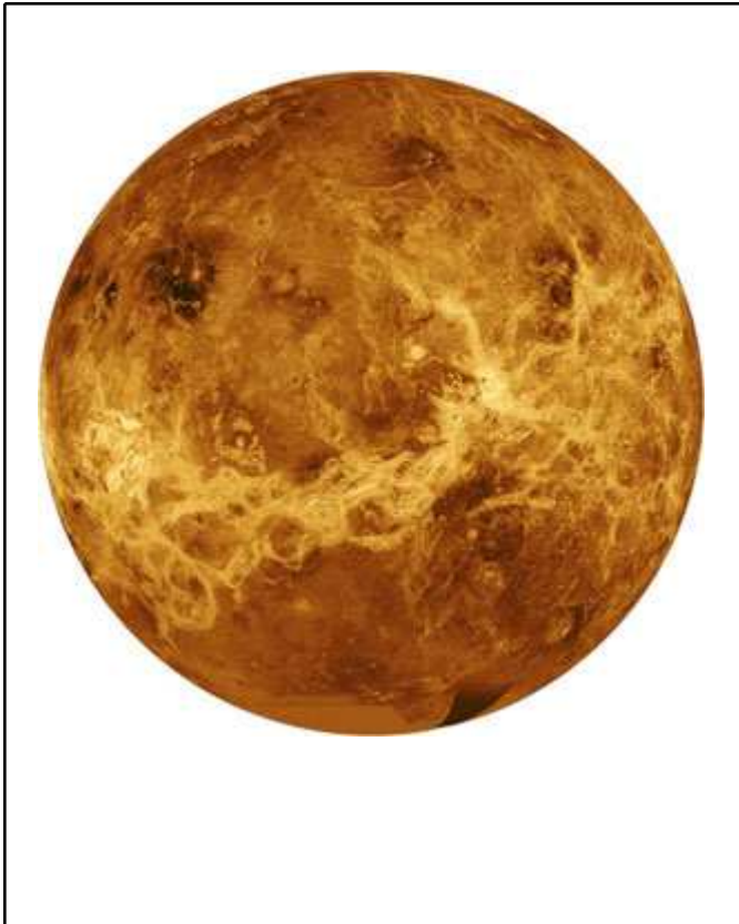
venus
